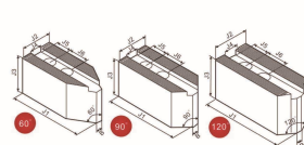
型號 / Model 重量 / Weight 螺絲 / Screw 尺寸 / Size (mm) 單位 / UNIT kg J1 J2 J3 J4 J5 J6 B mm SC08H3BP 2.5 38 SC08H6BP 3.2 60 SC08H6BP 3.8 60 SC08H7DP 4.4 M12 95 35 70 14 15 25 3 SC08H9DP 5.1 80 SC08H9DP 5.8 90 SC08H10DP 6.4 100
